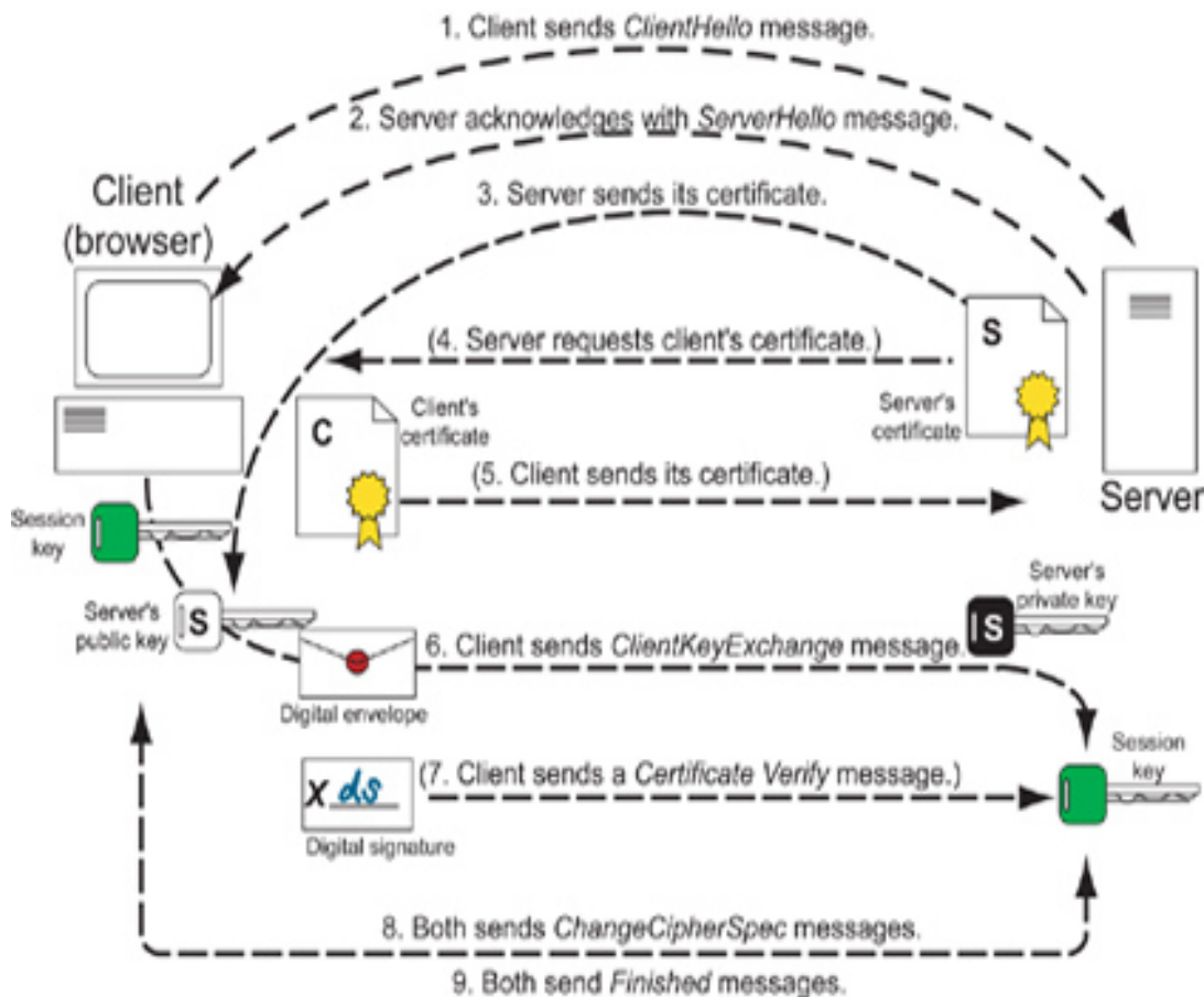
Fig. 2 - SSL Layer
